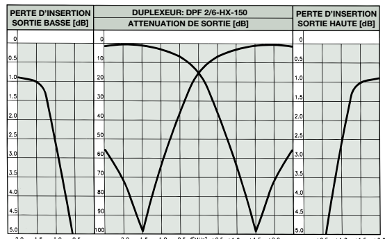
COURBES DE REPONSE TYPQUES ECART DUPLEX @ 3 MHz:
