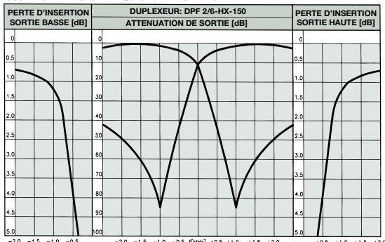
COURBES DE REPONSE TYPQUES ECART DUPLEX @ 2 MHz:
