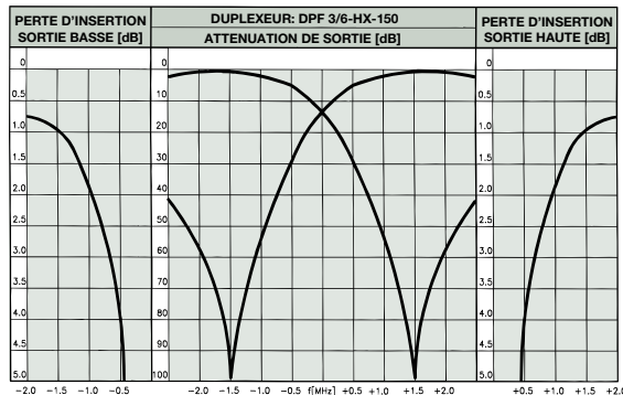
COURBES DE REPONSE TYPIQUES ECART DUPLEX @ 3 MHz:
