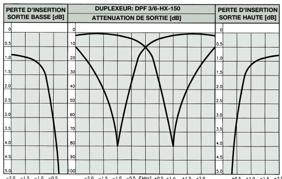
COURBES DE REPONSE TYPIQUES ECART DUPLEX @ 2 MHz:
