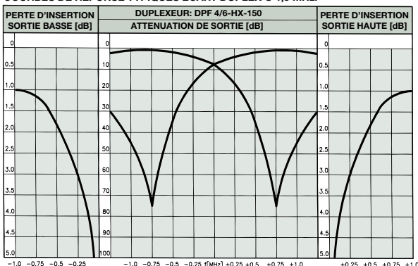
COURBES DE REPONSE TYPIQUES ECART DUPLEX @ 1,5 MHz:
