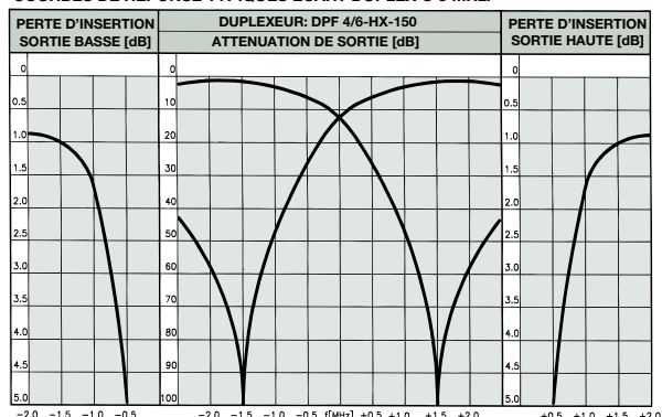
COURBES DE REPONSE TYPIQUES ECART DUPLEX @ 3 MHz:
