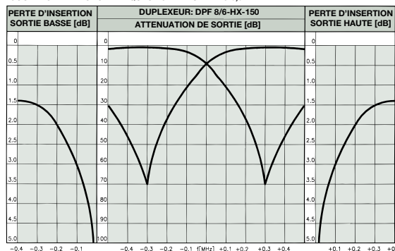
COURBES DE REPONSE TYPIQUES ECART DUPLEX @ 1,5 MHz:
