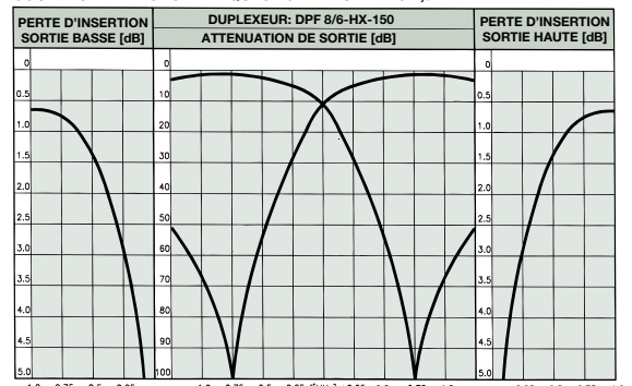
COURBES DE REPONSE TYPIQUES ECART DUPLEX @ 1,5 MHz:
