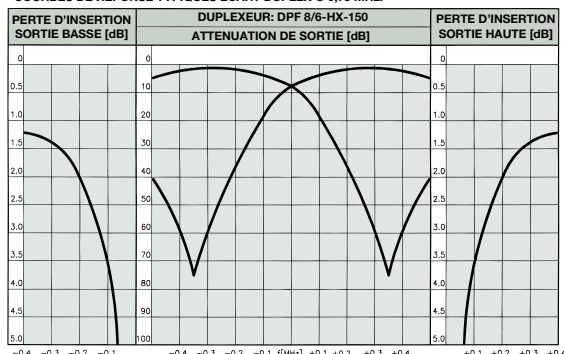
COURBES DE REPONSE TYPIQUES ECART DUPLEX @ 0,75 MHz:
